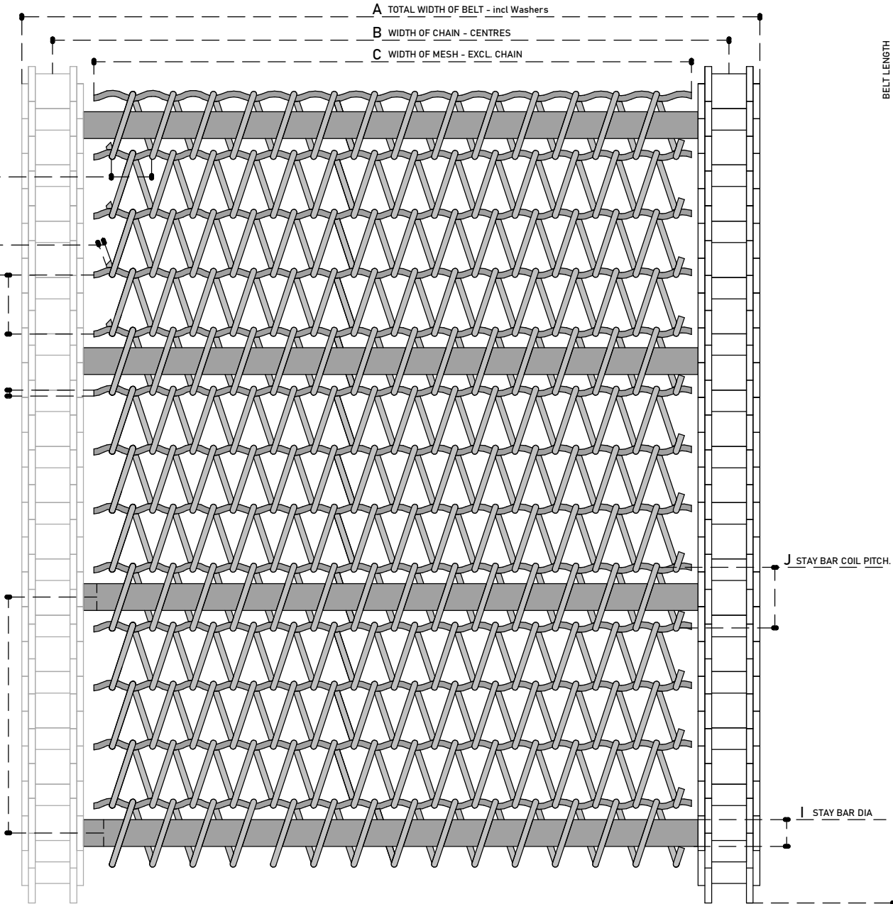
COTTERED EDGE
