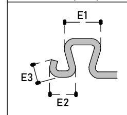
EDGE DETAIL : E1 / E2 / E3
